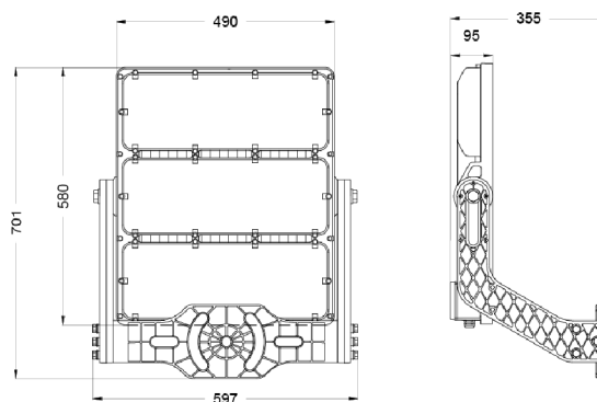
FLZ1K0A / FLZ1K2A / FLZ1K0B / FLZ1K2B
