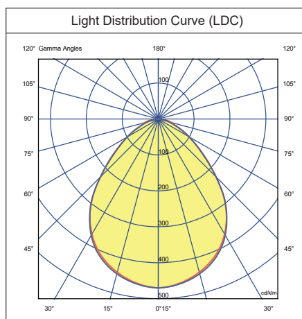
FPU435W4K-C
