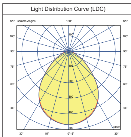
FPU435W4K-Z
