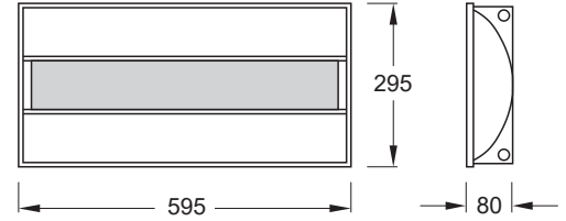
NUD2 - 600x300 mm
