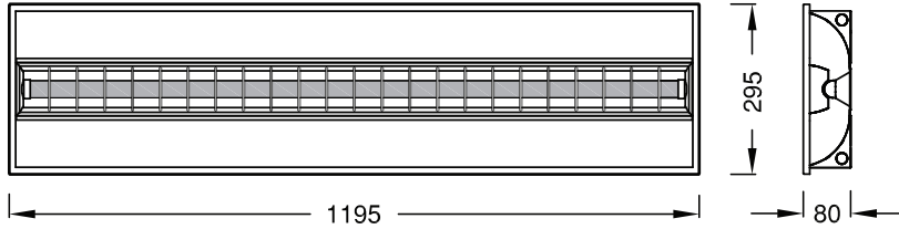
NUL4 - 1200x300 mm
