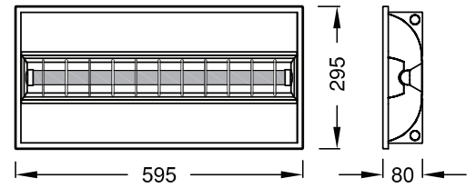
NUL2 - 600x300 mm
